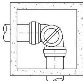
C - Raccordo angolare con innesto e curva aperta
