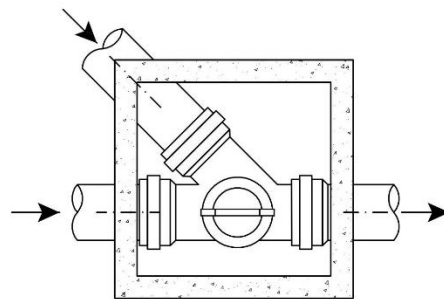
C - Raccordo angolare con innesto e curva aperta
