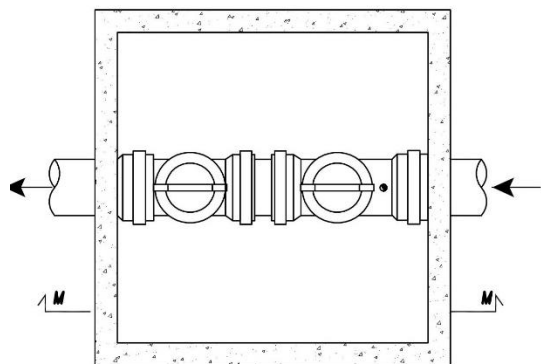
A - Sifone tipo Firenze
